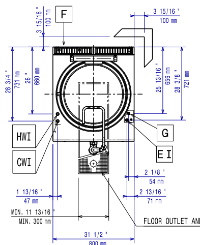
Boven aanzicht
